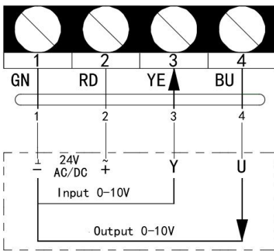
M 型接线图
