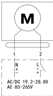
D 型接线图
