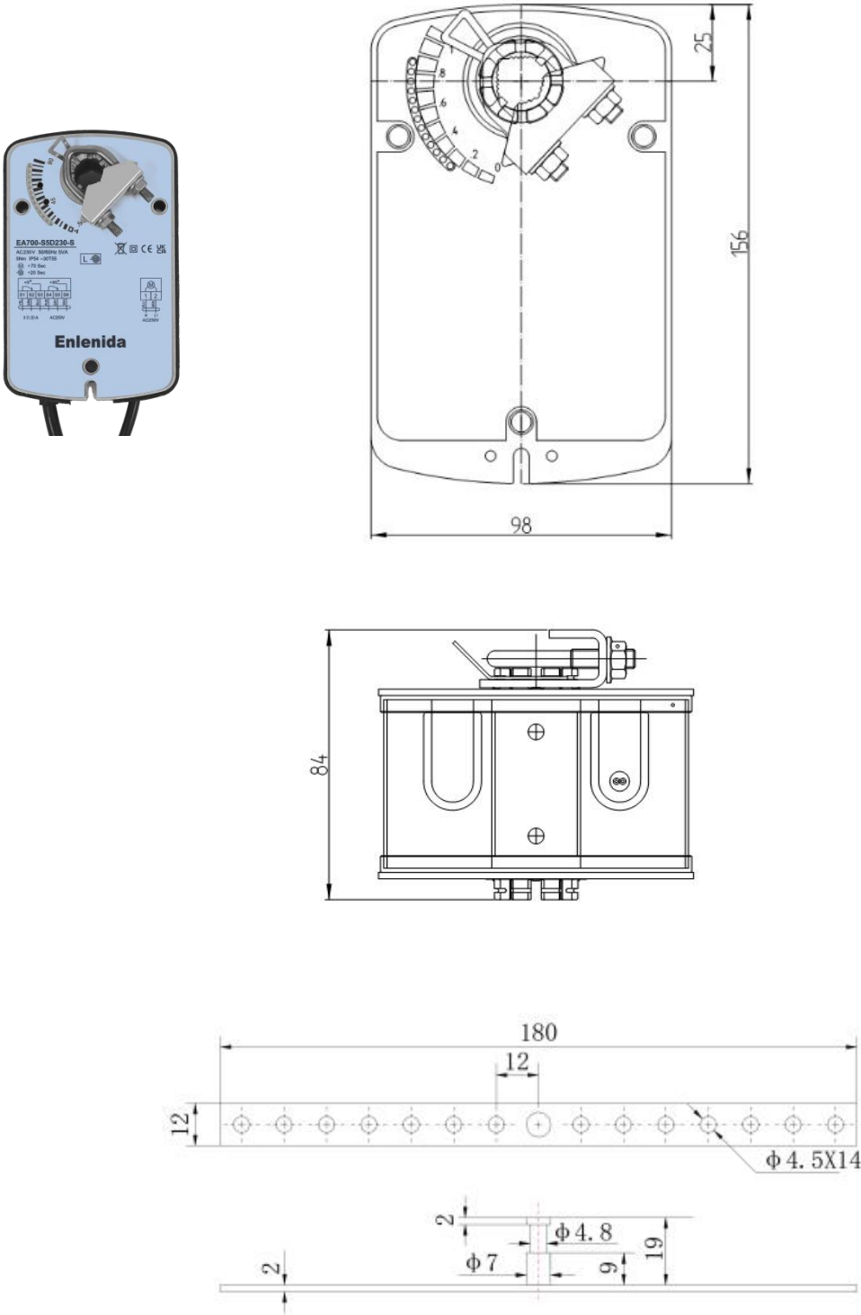
EA700-S5 外形及安装尺寸 单位 (mm)
