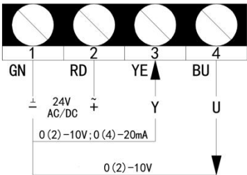
M 型接线图
